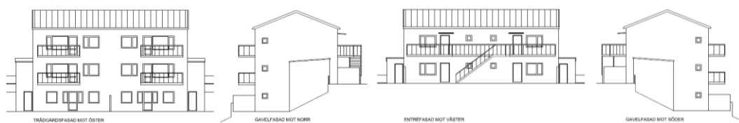
Fasader på ett av de föreslagna suterränghusen
