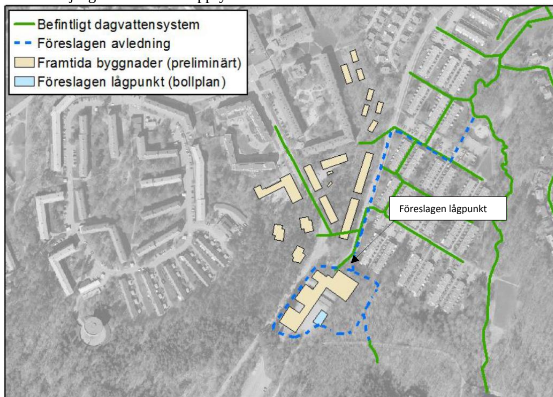
Planöversikt med föreslagna åtgärder i skyfallsutredningen
